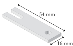
Distans till takmontering - Sidodrag/motor (standardbeslag)
