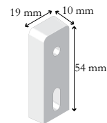
Distans, 10 mm För 70 mm
