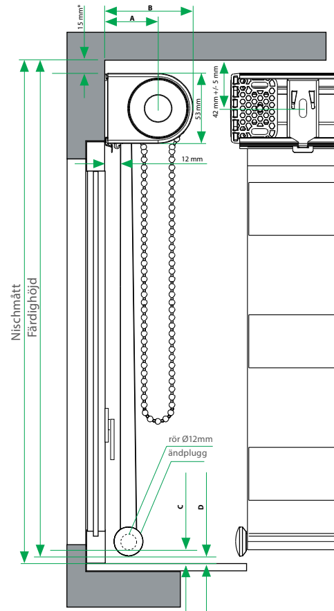
Vägg – monteringsprofil
