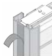
Ⓐ1 U-list med tejp och vinkel. Till modell 3242 levereras vinkel tillsammans med wirefot. Sidolisten kan också monteras på glas.
