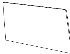
SA350 kupévägg höger/vänster (19) H 1315 B 2440 D 45
