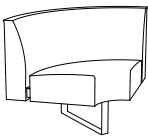
SA640 H 795 SH 450 B 815 D 815
