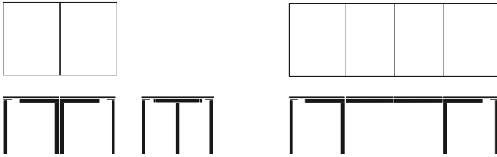
1600 × 900 mm + två st iläggsskivor à 500 mm, H 720 mm
