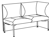
SA820 fristående (8) H 850 SH 450 B 1295 D 665
