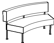
SA2250 H 780 SH 450 B 1470/1960/2450 D 600
