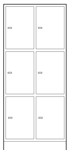
SD8/19 1932 x 800 x 580
